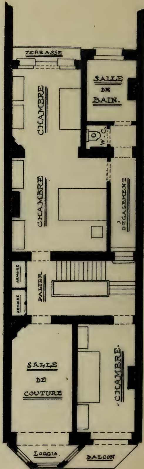
1er ÉTAGE
